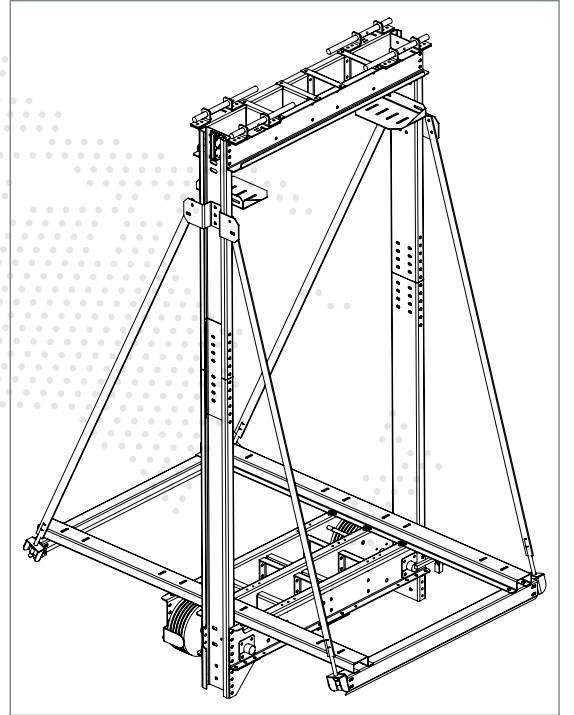
MRL Süspansiyon 1600 2000 Kg. Machine roomless suspension 1600 2000 Kg.
