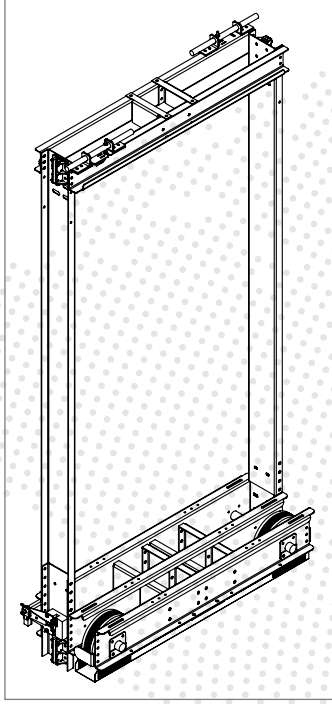
MRL Yandan Ağırlık - Süspansiyon Machine roomless elevator with side weight suspension
